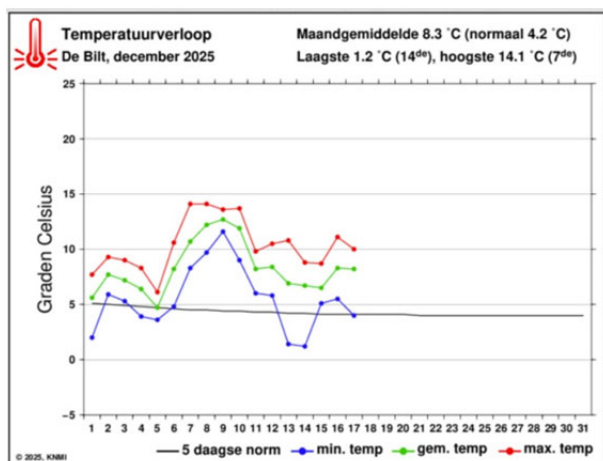
KNMI: Temperaturen per dag 1 t/m 17 dec 2025
